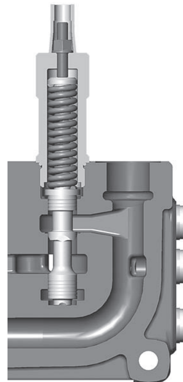
PLS – Begrenzungsfunktion zur Einstellung der Druckdifferenz zwischen Pumpendruck und Lastsignal.
