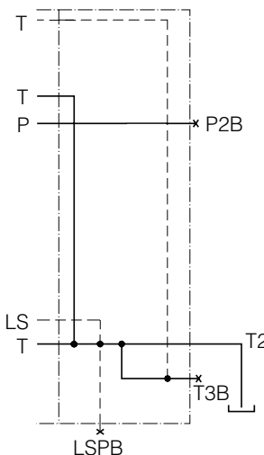
T2 – Ohne Gegendruckventil.
