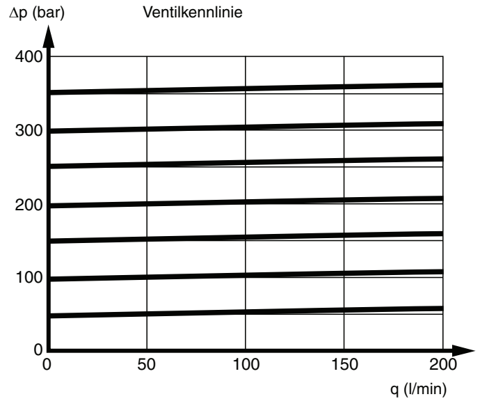
PS - Vorgesteuertes Druckbegrenzungsventil
