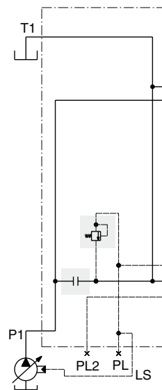
AS2 – Eingangssektion für das zweite Ventil in einem Stromteilungssystem
