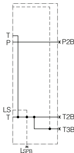
LSPB – LSP-Anschluss intern mit dem Tankkanal verbunden.
