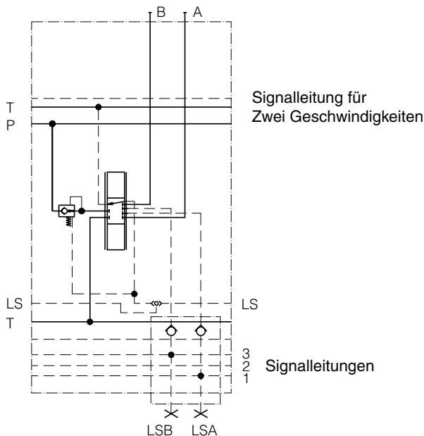
SF – System-Signalleitung
