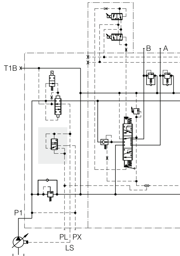
KS – Eingangssektion mit Kopierschieber
