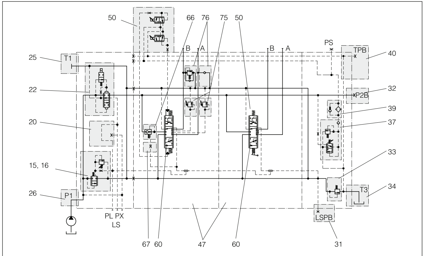
Hydraulikschaltbild mit Darstellung der Grundfunktionen für L90LS
