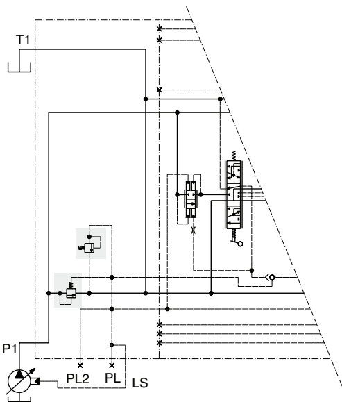
AS – Eingangssektion für das erste Ventil im Stromteilungssystem
