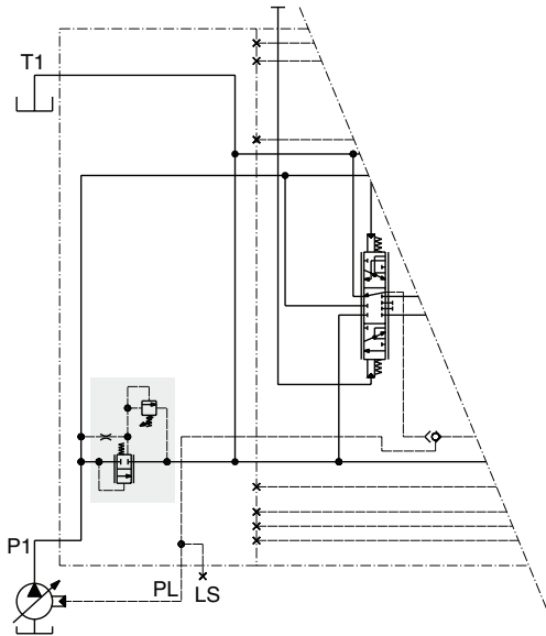
LS1 – Eingangssektion für Systeme mit Verstellpumpe
