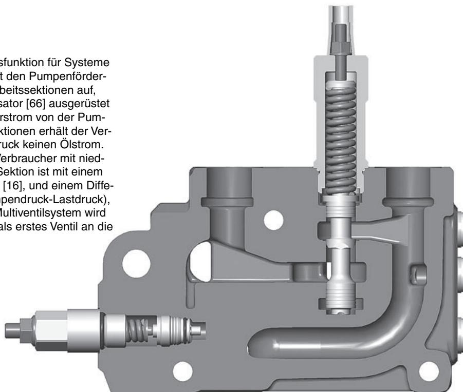
Eingangssektion AS
