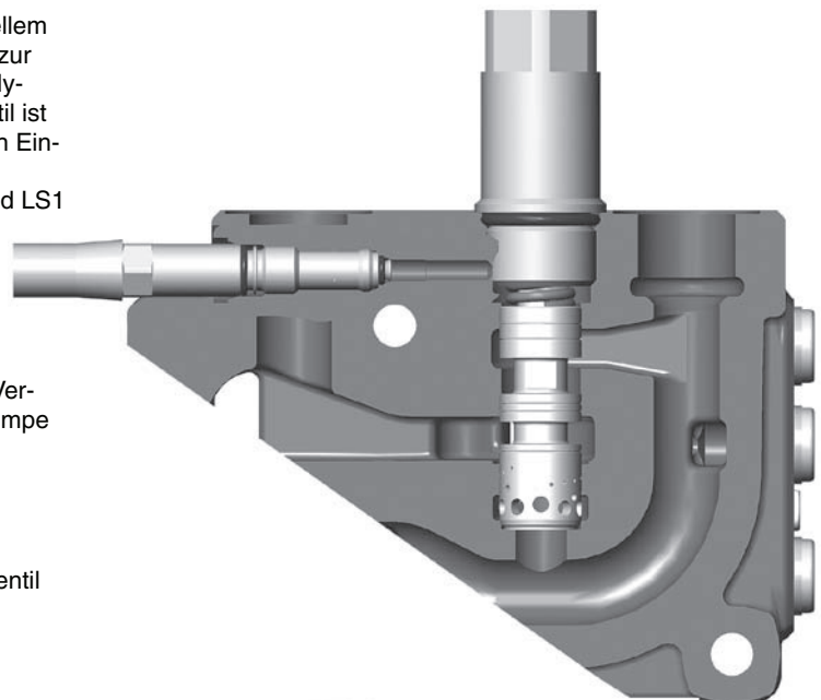
PS – Vorgesteuertes Druckbegrenzungsventil für Eingangsektion CFC und LS1.
