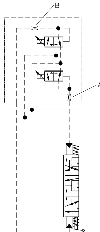
Steuerdruck-Drosselung
