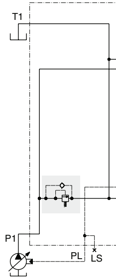
LS2 – Eingangssektion für Systeme mit Verstellpumpe
