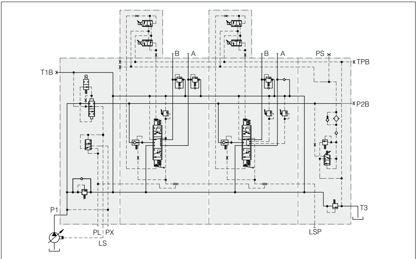
L90LS mit elektrohydraulischer Betätigung, ausgerüstet mit direktgesteuertem Hauptdruckbegrenzungsventil für Systeme mit Verstellpumpe, Pumpenentlastungsfunktion, integrierter Steueröl-
