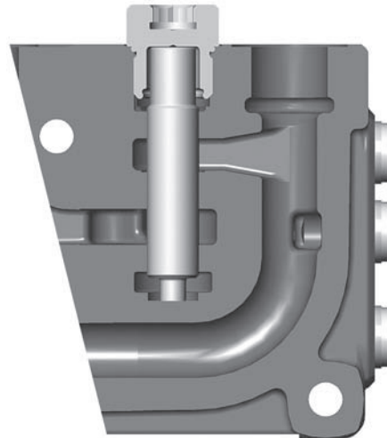
Eingangssektion AS2
