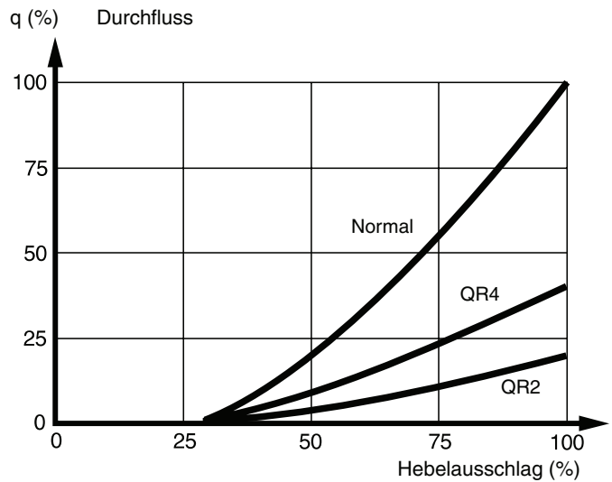
Das Diagramm enthält die Kurven: Normaler Durchfluss Durchfluss bei Aktivierung von QR4 Durchfluss bei Aktivierung von QR2
