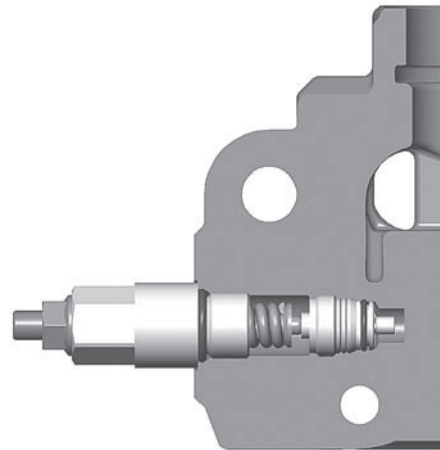
PLM – Druckbegrenzungsventil für Eingangsektion AS und AS2.
