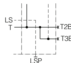
LSP – Anschluss des Lastsignals für ein anderes Ventil geöffnet.
