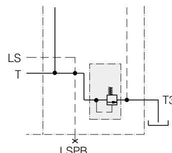
MF – Fest eingestelltes Gegendruckventil.
