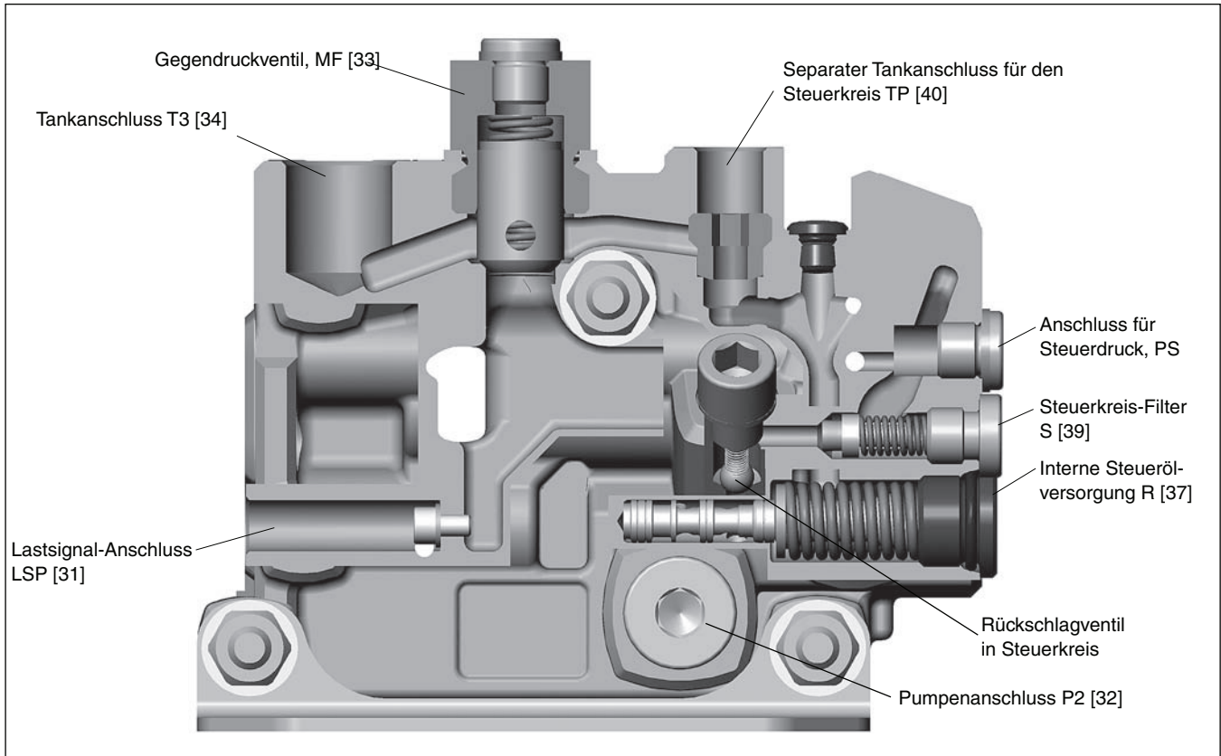
Endsektion US mit Steuerölversorgung, Steuerkreis-Filter, Gegendruckventil und separater Tankanschluss für den Steuerkreis
