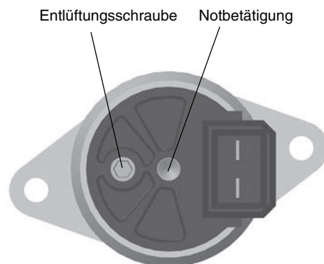
EC-Vorsteuermagnetventil mit Notbetätigung und Entlüftung.
