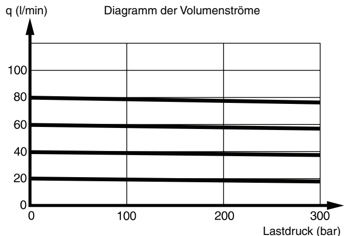
Lastabhängiger Durchfluss mit Druckwaage.
