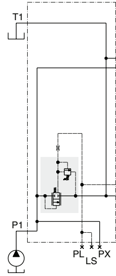
CFC – Eingangssektion für Systeme mit Konstantpumpe
