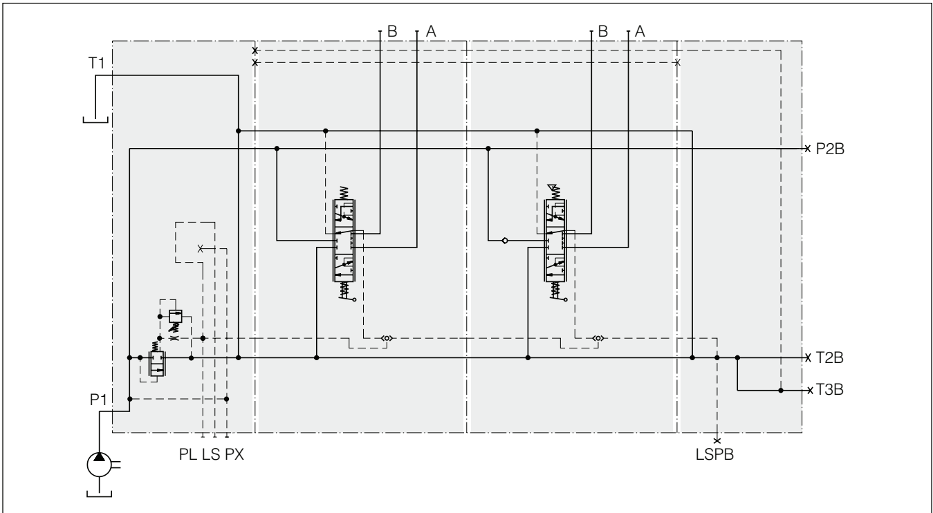
L90LS handbetätigt, ausgerüstet mit 3-Wege-Druckwaage für Konstantstromsysteme.
