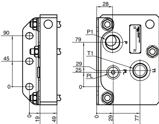
Eingangssektion IP
