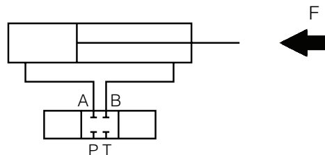
LA - Hebelast normalerweise nur am A-Anschluss.
