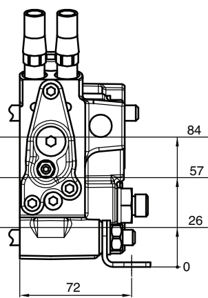
Schieber-Endsektion MU
