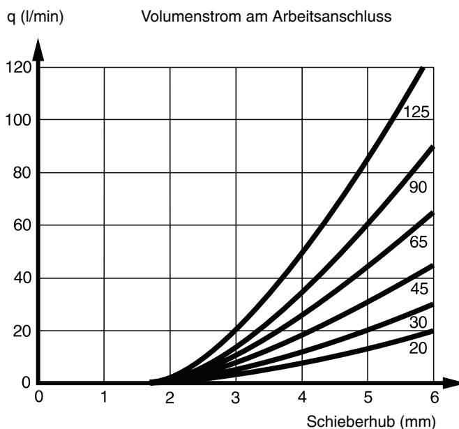
Durchfluss als Funktion des Schieberhubs bei verschiedenen Ausführungen
