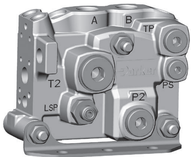
Kombinierte Schieber- und Endsektion, MU.
