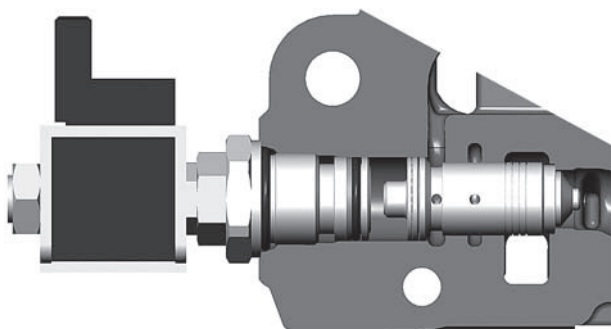
BEN – Elektrisch betätigte Pumpenentlastungsfunktion
