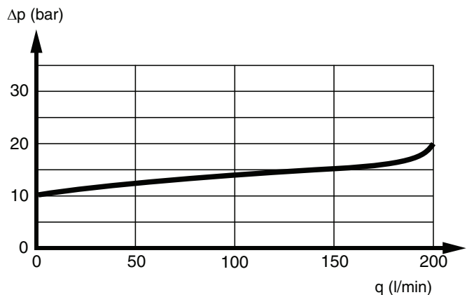
CFC – Leerlauf-Druckabfall im der Bypass. P1 - T1
