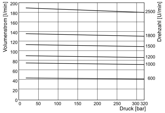
P2145 Volumenstrom - voller Hub
