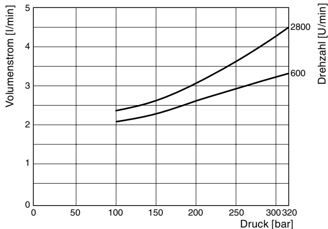
P2105 Pumpenlecköl bei Nullhub
