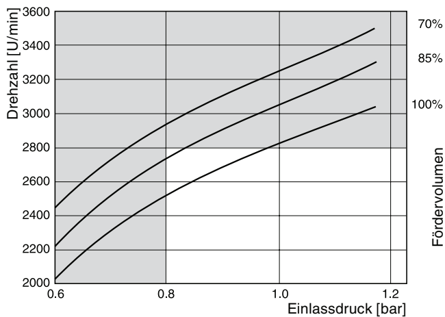
P2105 Eingangskenngrößen
