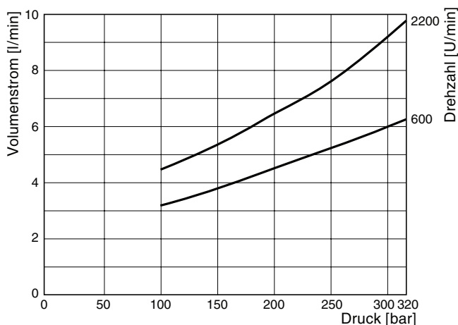
P2145 Pumpenlecköl bei Nullhub
