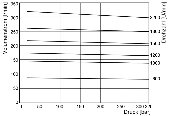
P2145 Volumenstrom - voller Hub
