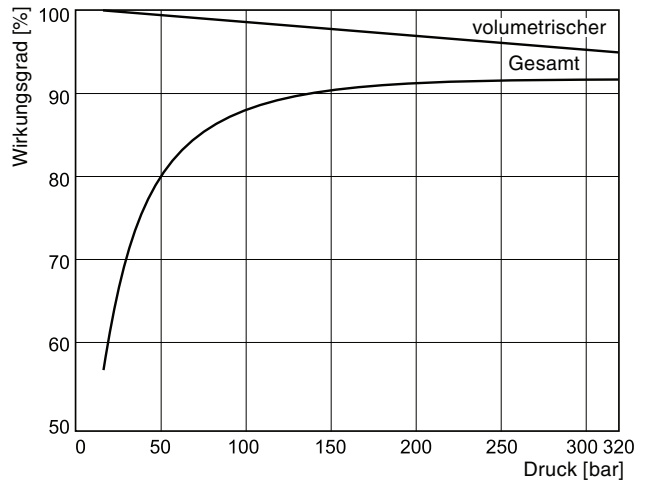
P2145 Wirkungsgrad bei 1800 U/min
