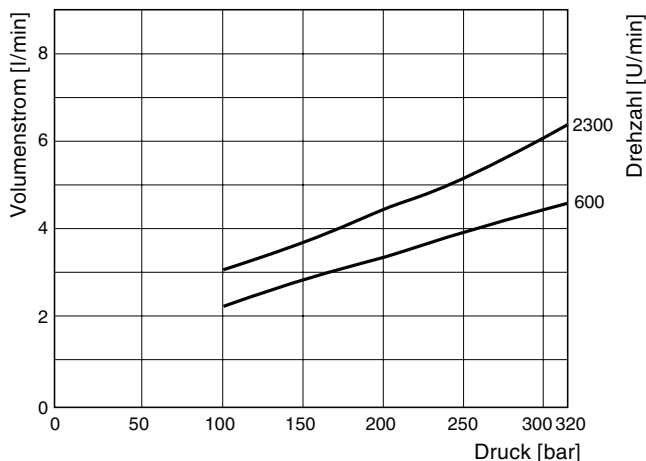
P2105 Pumpenlecköl bei Nullhub
