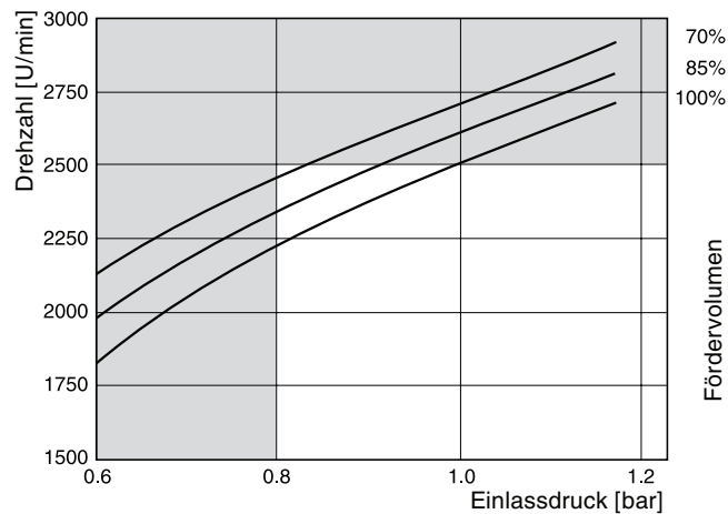
P2145 Eingangskenngrößen
