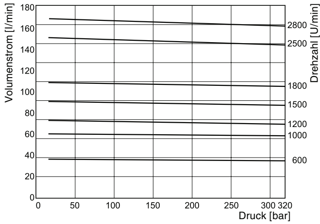
P2105 Volumenstrom - voller Hub
